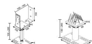
Brides latérales-R
